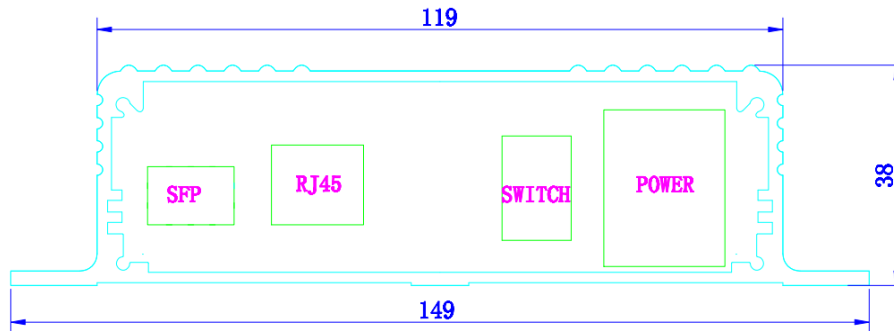
Fig. 1 CVT310 external dimensions
