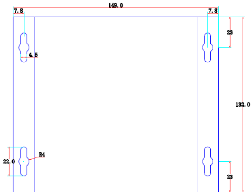
Fig. 3 CVT310 positioning
