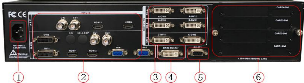
图 1—视频处理器后面板
