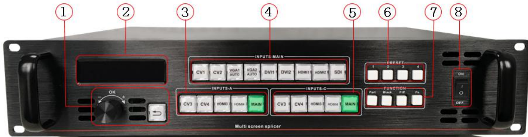
图3—处理器前面板
